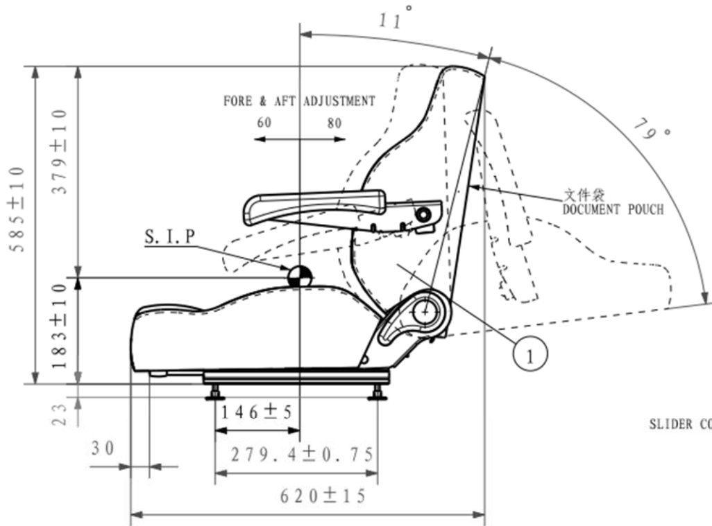
VIEW A-A
